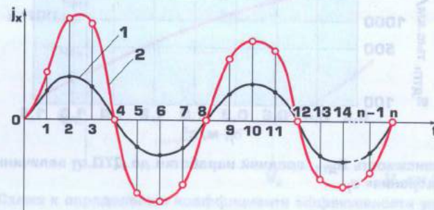
Рис. 7.1. Схема к определению среднеквадратичного отклонения \sigma_j величины продольного ускорения автомобиля:
