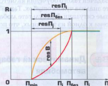
Рис. 6.3. Изменение надежности управления R в зависимости от величины параметра пространства \Pi при постоянной скорости V_a :
