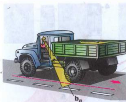
Рис. 4.4. Контроль траектории автомобиля при движении задним ходом по величине левого интервала b_n
