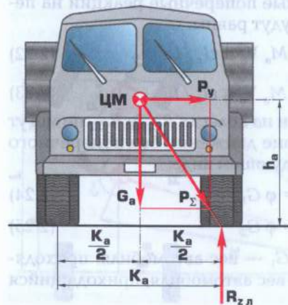
Рис. 2.5. Силы, действующие на автомобиль в момент опрокидывания:
