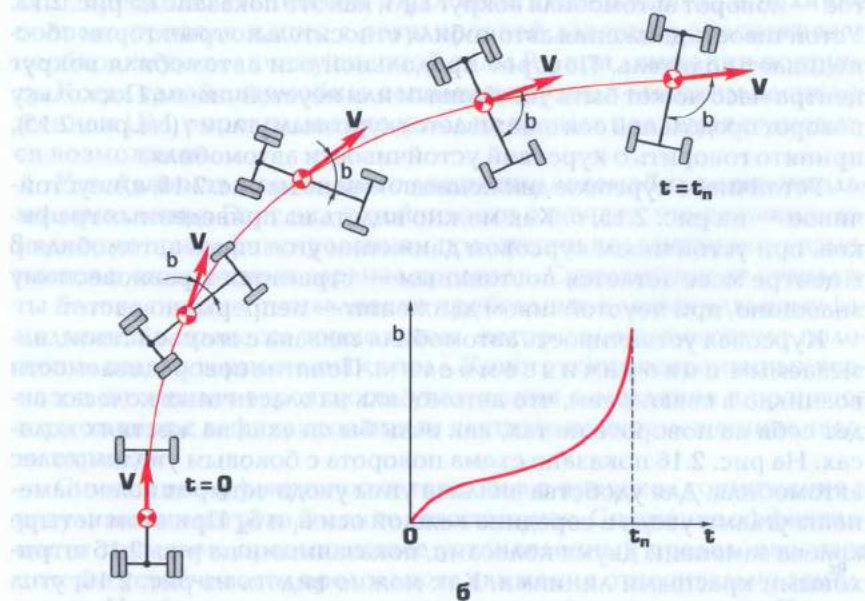
Рис. 2.15. Определение условий сохранения курсовой устойчивости автомобиля:
