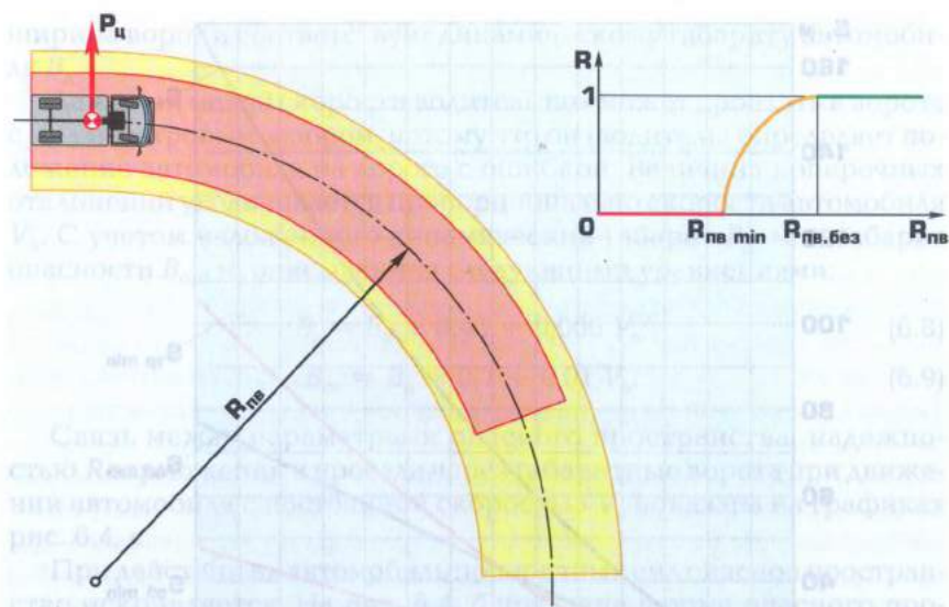
Рис. 6.6. Искривление опасного пространства при повороте автомобиля:
