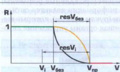
Рис. 1.5. Определение резерва скорости и зависимости надежности управления от величины резерва:
