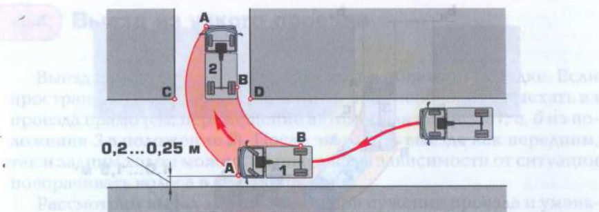
Рис. 4.9. Въезд передним ходом в узкий проезд, расположенный на прилегающей стороне дороги:
