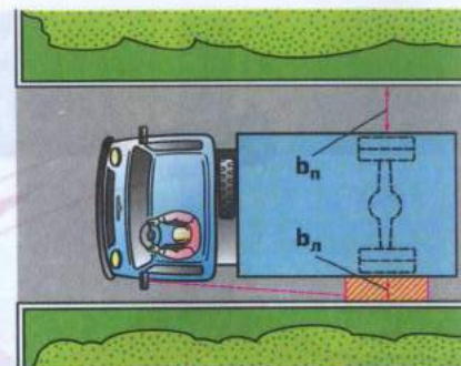
Рис. 4.5. Уменьшение левого интервала b_n и увеличение правого интервала b_n в узких проездах
