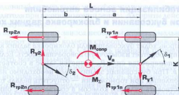
Рис. 5.11.1. Схема движения автомобиля при неравномерном распределении реакций торможения R_{тр} по бортам автомобиля:
