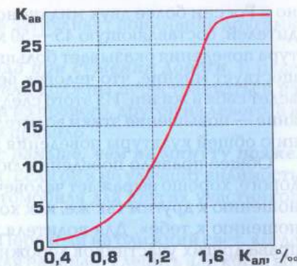
Рис. 1.14. Зависимость коэффициента аварийности K_{ав} от концентрации алкоголя в крови K_{ал}
