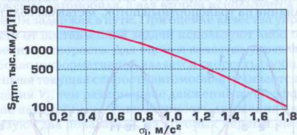
Рис. 7.2. Зависимость S_{\text{ДТП}} средней наработки до ДТП от величины «шума ускорения» \sigma_j
