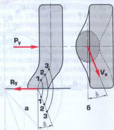
Рис. 2.8. Схема бокового увода колеса:
