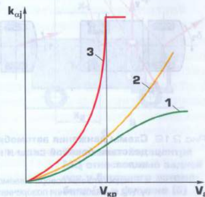
Рис. 2.18. Изменение чувствительности к повороту рулевого колеса автомобилей с разной поворачиваемостью в зависимости от скорости:
