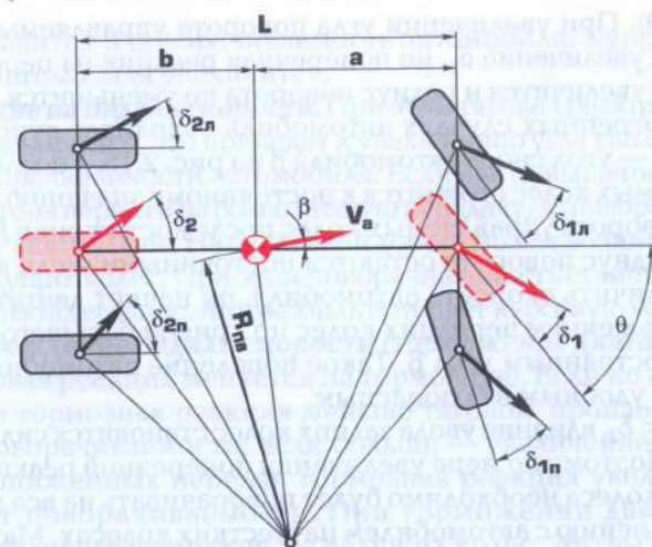
Рис. 2.16. Схема поворота автомобиля с боковым уводом колес
