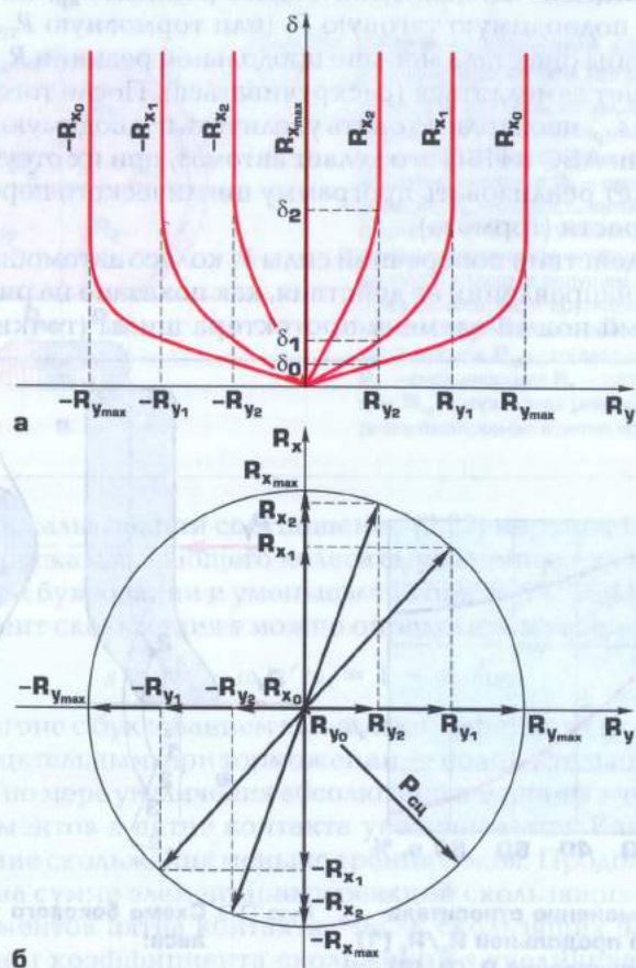
Рис. 2.9. Характеристики увода и скольжения колеса:
