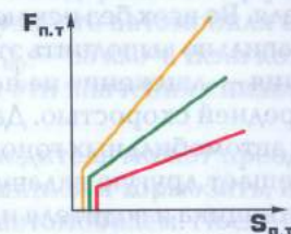
Рис. 3.19. Характеристики «жесткости педали тормоза», т. е. зависимости усилия перемещения педали F_{п.т} от величины ее перемещения S_{п.т} :
