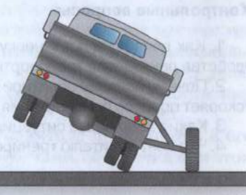
Рис. 10.4. Выполнение маневра «поворот» с опрокидыванием автомобиля на страховочное приспособление
