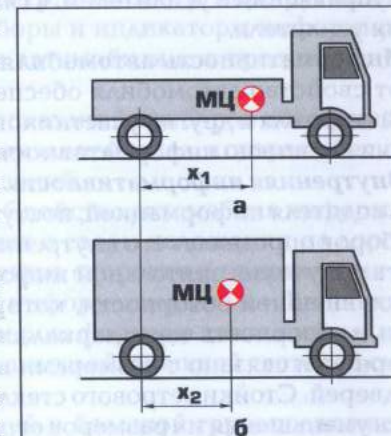
Рис. 2.20. Положения метacentра МЦ относительно задней оси у бортового автомобиля (а) и фургона (б)
