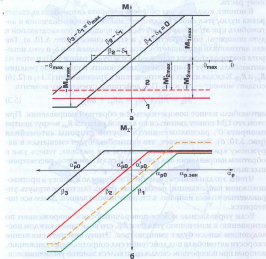
Рис. 5.9. Зависимость изменения моментов, действующих на автомобиль, от угла поворота управляемых колес \theta (рулевого колеса \alpha_p ) при различных углах сноса \beta :
