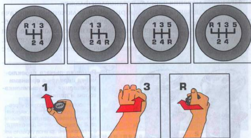
Рис. 3.4. Схемы переключения четырех- и пятиступенчатых коробок передач
