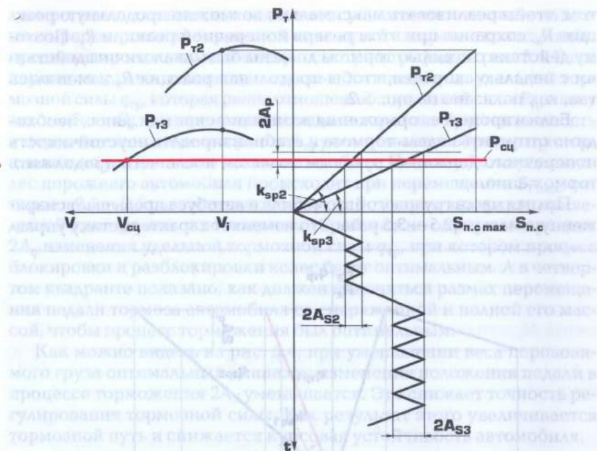
Рис. 5.3. Влияние выбранной передачи на размахи перемещения педали скорости 2A_S при движении с буксованием ведущих колес:
