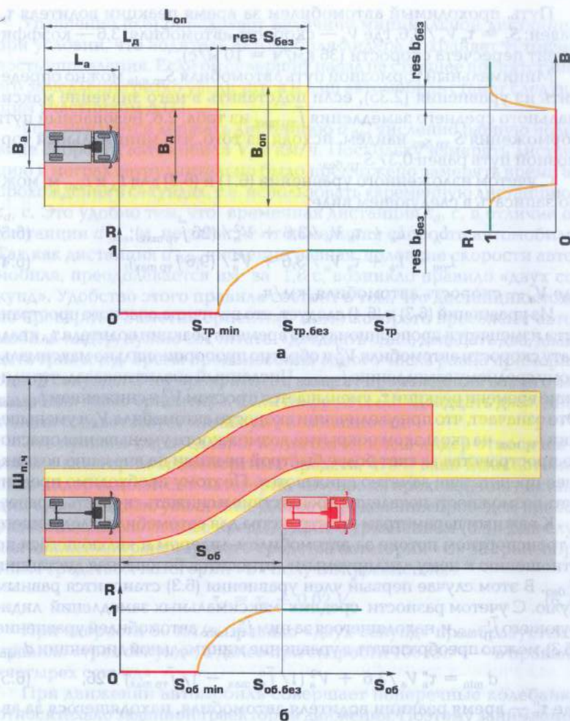
Рис. 6.4. Опасное пространство, возникающее вокруг автомобиля:
