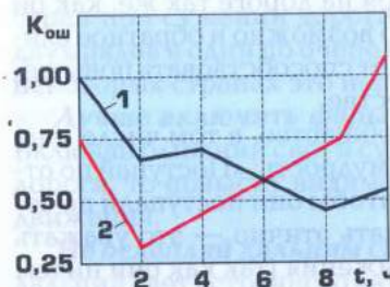
Рис. 1.13. Зависимость относительного показателя числа ошибок K_{ош} от времени t при исследовании сложных сенсомоторных реакций:
