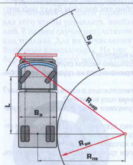
Рис. 4.1. Увеличение габаритной ширины автомобиля на повороте:
